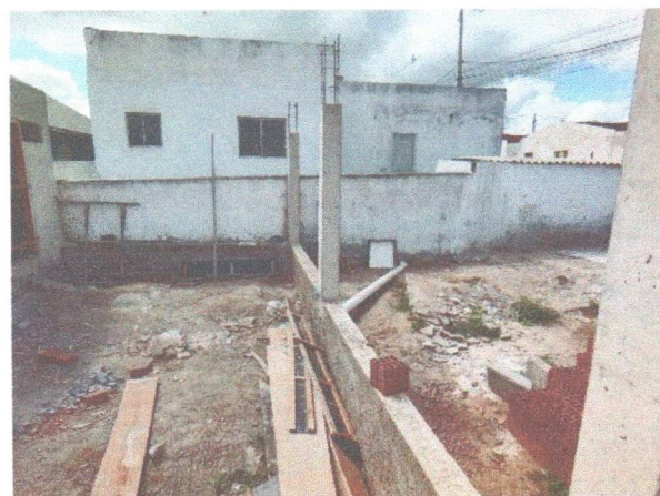
FOTO 3: Pilares da Coberta e Contenção do aterro;
