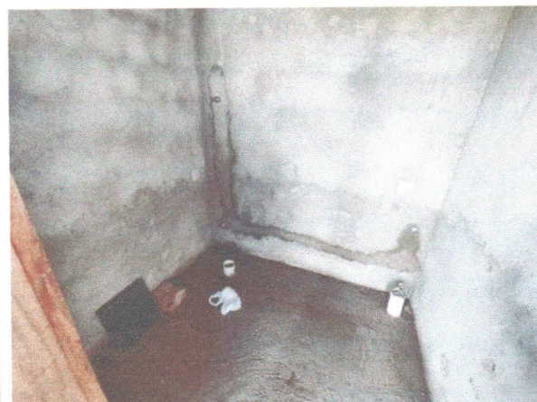
FOTO 5: Lastro de piso e pontos de esgoto;
