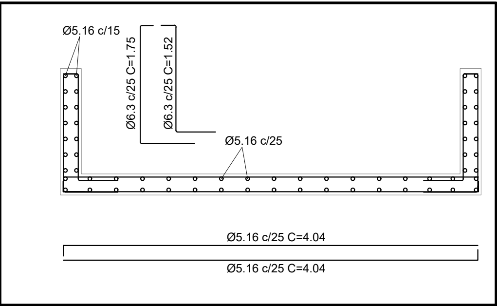
2 DETALHE DA ARMAÇÃO ESCALA 1:35
