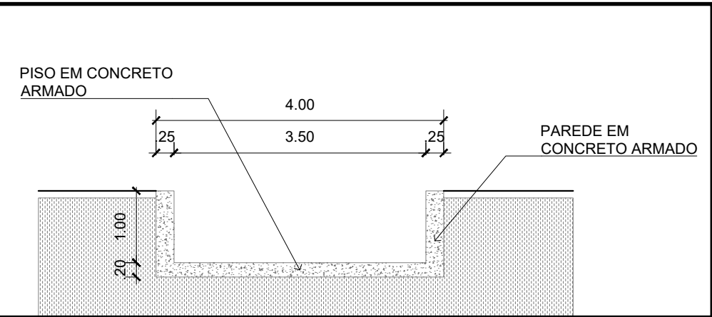
2 PERFIL DO CANAL ESCALA 1:75
